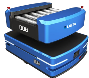
LISTA Roller mit Rollenband-Aufbau für leichteres Be- und Entladen
